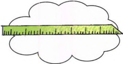
مسطرة
